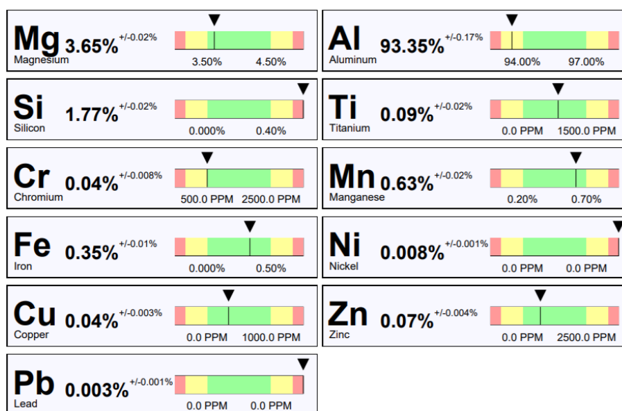
Slika 40. Rezultati ispitivanja kemijskog sastava na mjereno području 4
