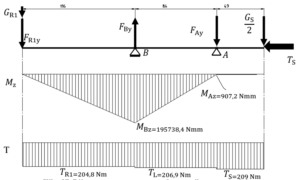
Slika 87. Dijagram momenata pogonskog vratila u x-y ravnini
