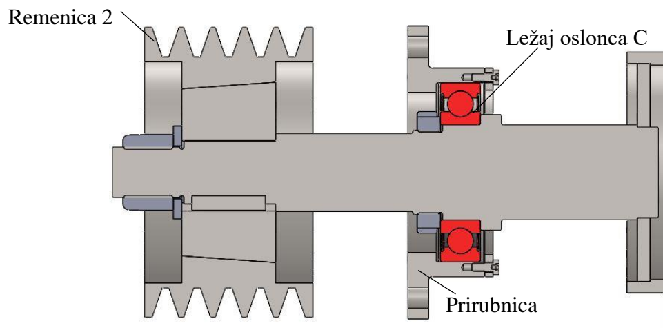
Slika 144. Vratilo 2
