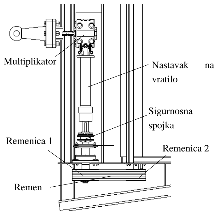
Slika 70. Prijenos snage koncepta 2
