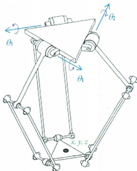
Slika 10. Delta robot dijagram, [8]
