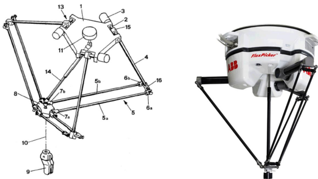
Slika 9. Dizajn iz Cavelovog patenta [6] (lijevo) i ABB-ov FlexPicker (desno)
