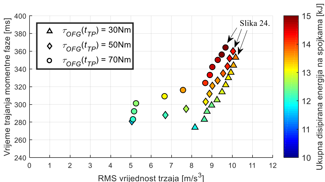
Slika 23. Performanse upravljanja bez kompenzacije izlaznog momenta za različite prijelazne momente OFG spojke \tau_{OFG}(t_{TP}) i različita trajanja momentne faze t_{TP} u slučaju zatvorenog pretvarača momenta
