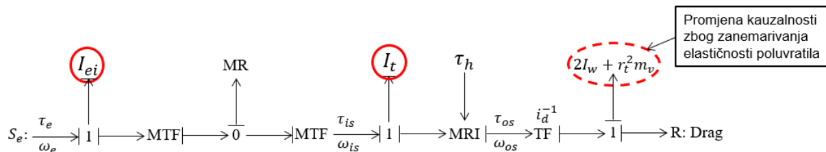
Slika 6. Vezni dijagram pogona vozila uz zanemareno uvijanje poluvratila
