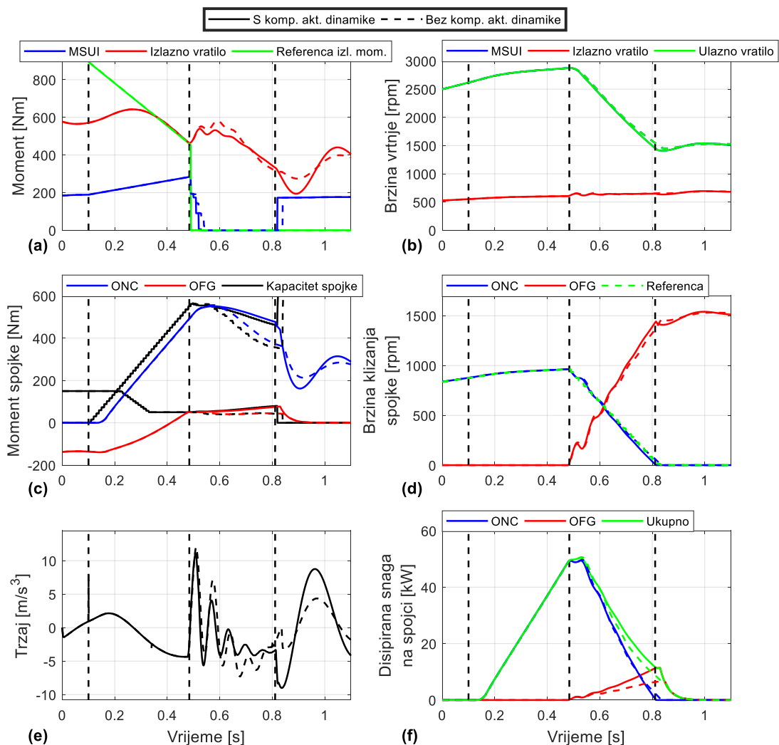
Slika 43. Simulacijski rezultati promjene stupnja prijenosa za LQR s i bez uključene kompenzacije aktuatorске dinamike, s kompenzacijom propada momenta na izlaznom vratilu transmisije za vrijeme momentne faze, t_{TP} = 350 ms, t_{IP} = 350 ms i zatvoreni pretvarač momenta
