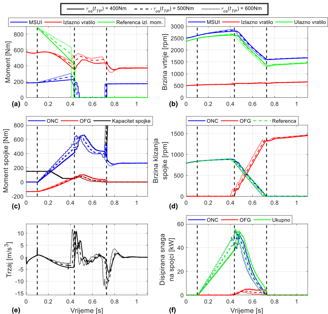
Slika 26. Simulacijski rezultati promjene stupnja prijenosa s obzirom na promjenu prijelaznog momenta izlaznog vratila \tau_{os}(t_{TP}) , željeno trajanje momentne faze t_{TP} = 350\text{ ms} i otvoreni pretvarač momenta
