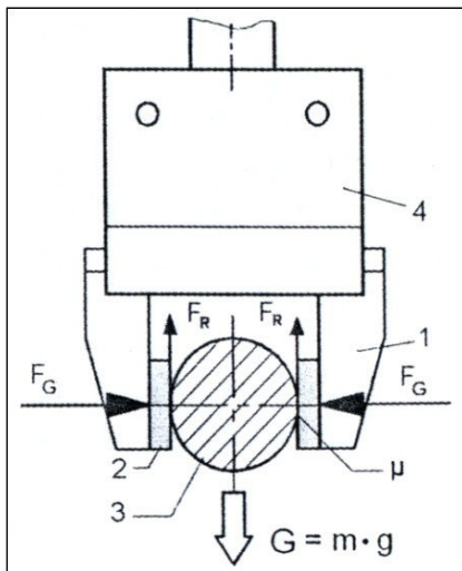
Slika 11. Schematski prikaz sile na prstima dvoprstne hvataljke [1]
