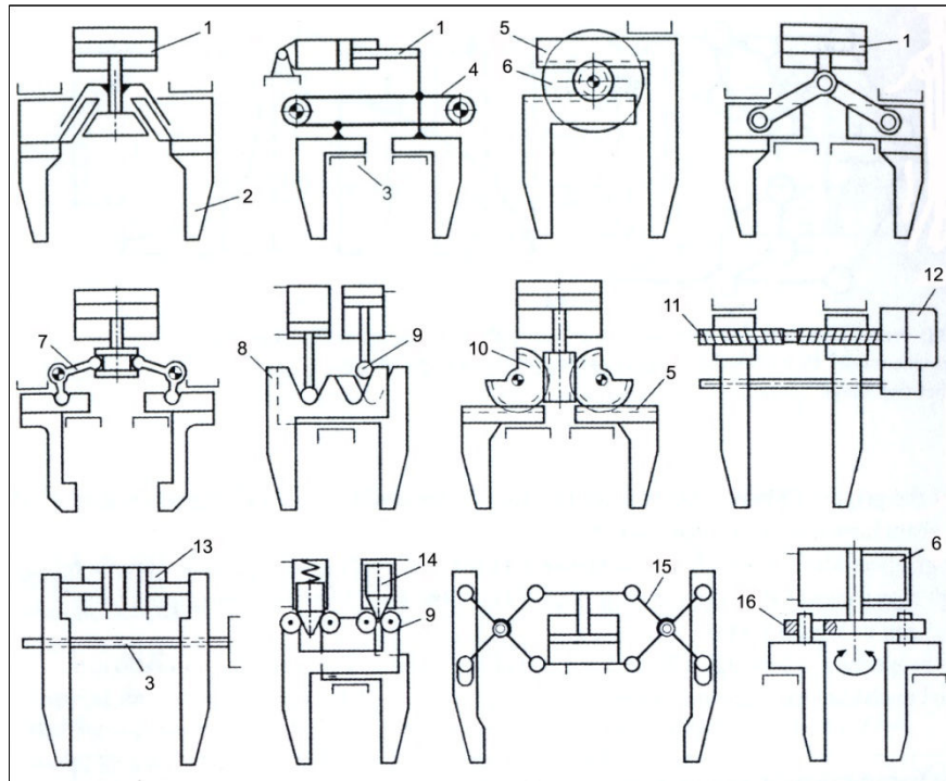
Slika 21. Shematski prikaz kinematskih modela translatorsnih stezних hvataljki [1]
