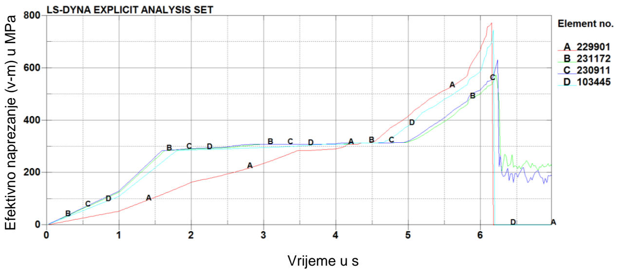
Slika 11-4 Dijagram ovisnosti vremena o napreznaju za 4 konačna elementa
