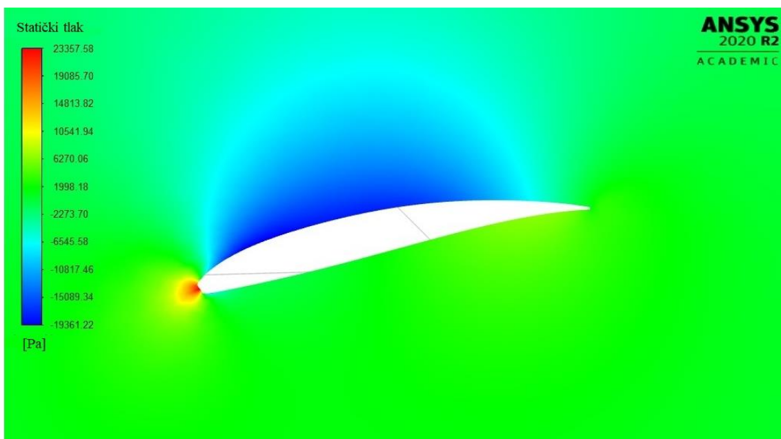
Slika 45. Polje statičkog tlaka oko poprečnog presjeka lopatice turbine bez statora na visini R = 0,9 m
