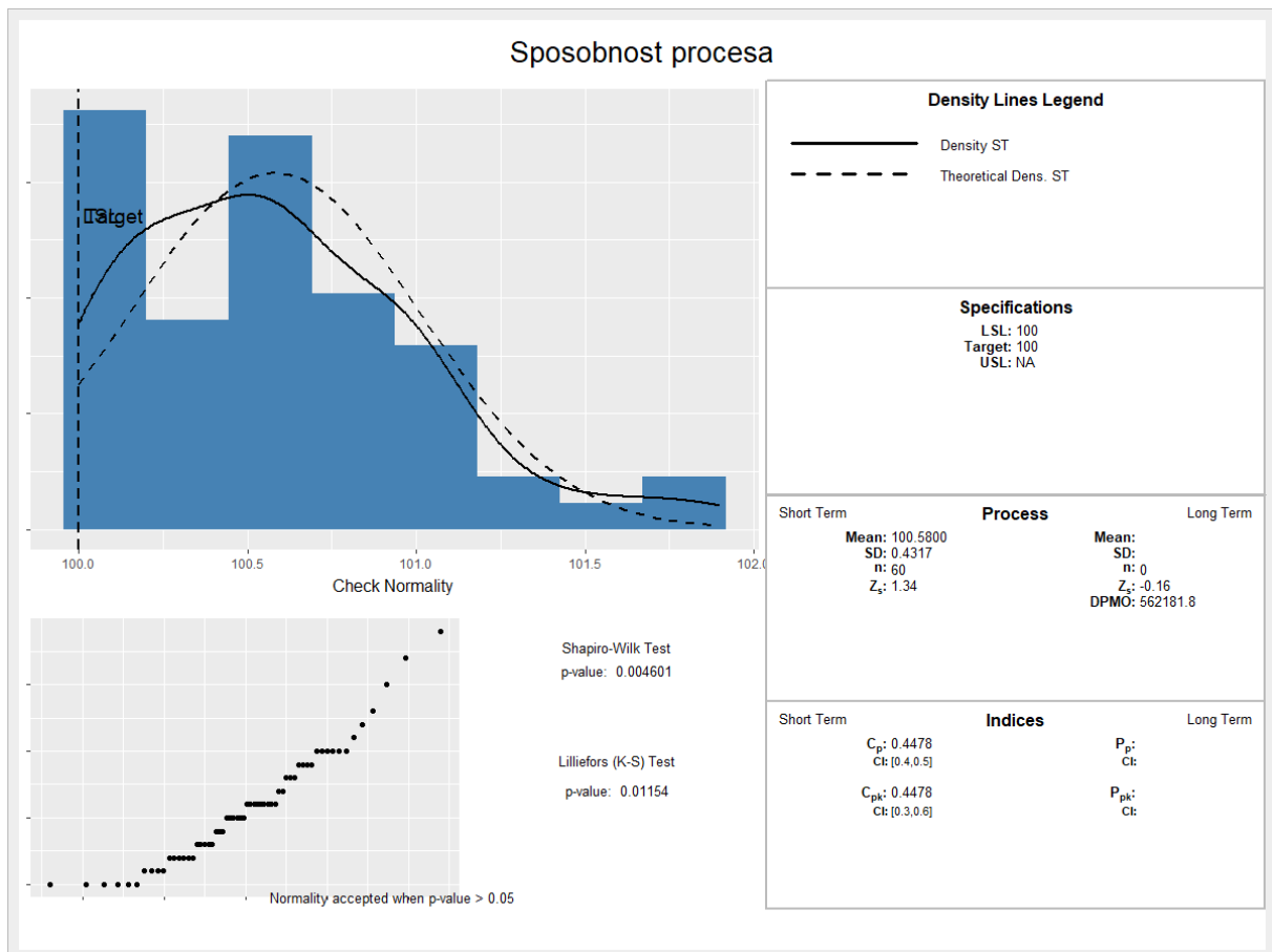
Slika 31. Sposobnost procesa
