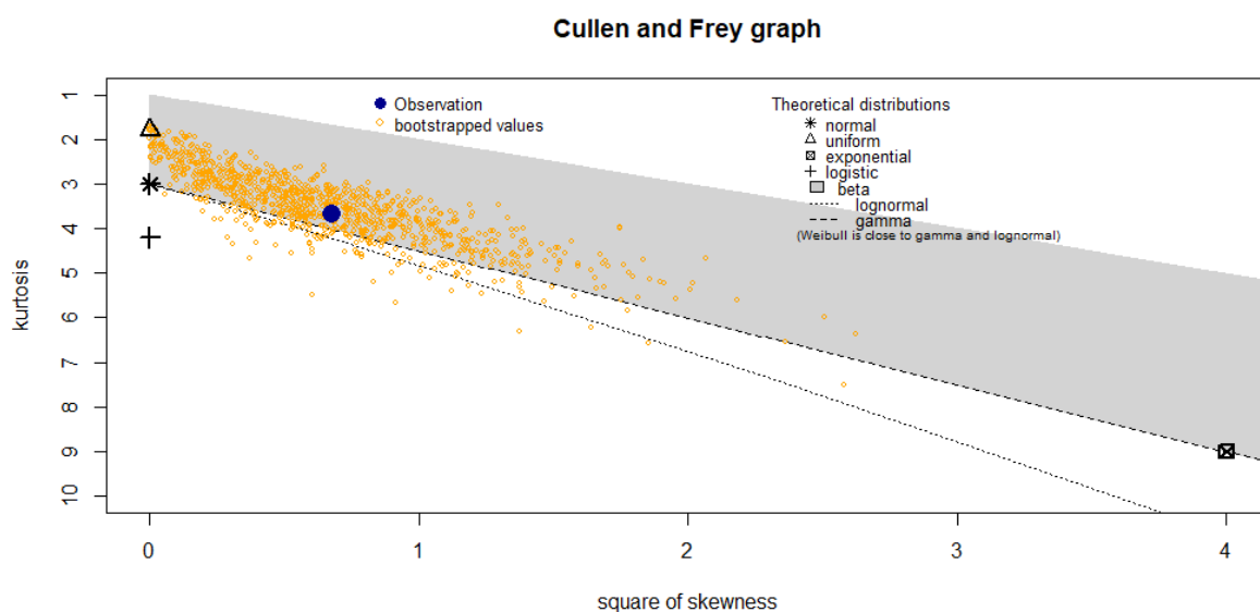
Slika 32. Cullen-Frey graf
