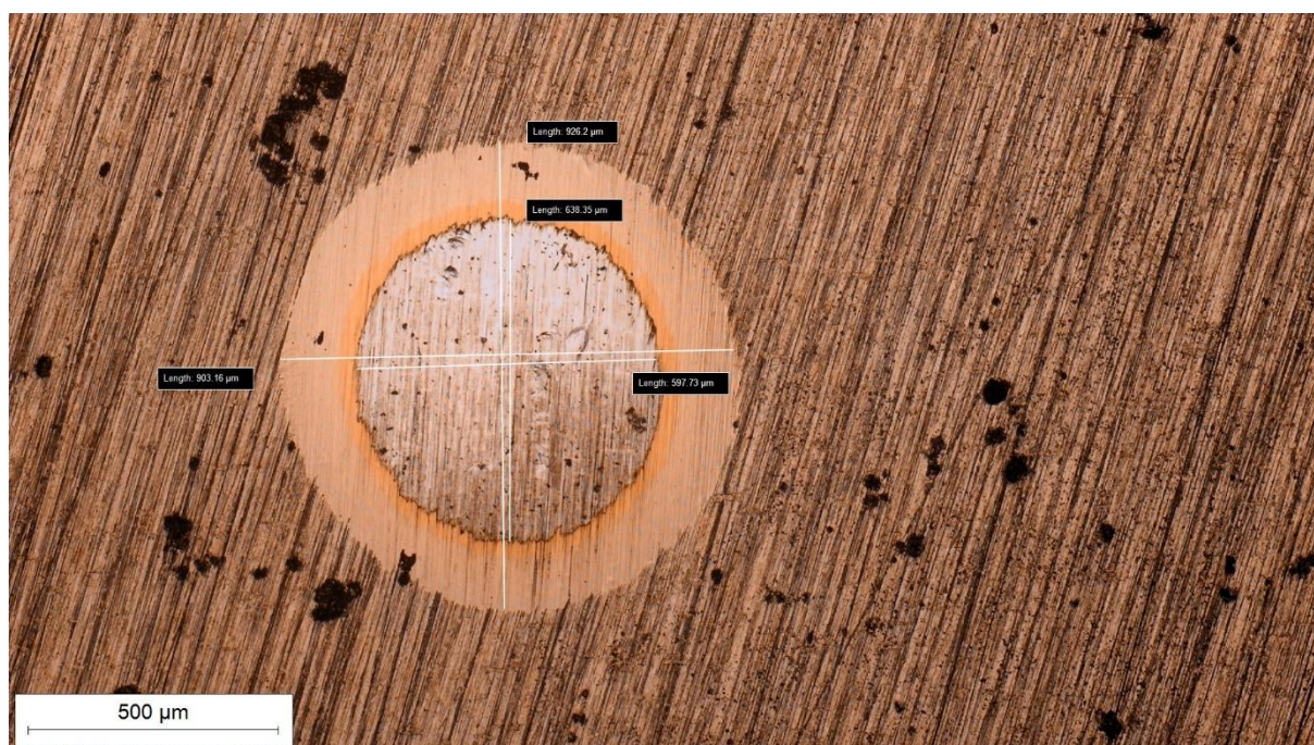
Slika 35. Trag trošenja na čeliku K110 snimljen na svjetlosnom mikroskopu nakon ispitivanja debljine prevlake metodom utiskivanja kuglice na uzorku D3 s TiN/TiBN prevlakom
