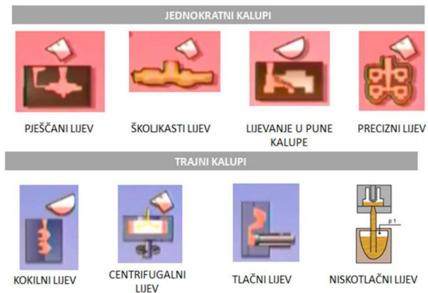
Slika 2. Podjela postupaka lijevanja prema vrsti kalupa [7]
