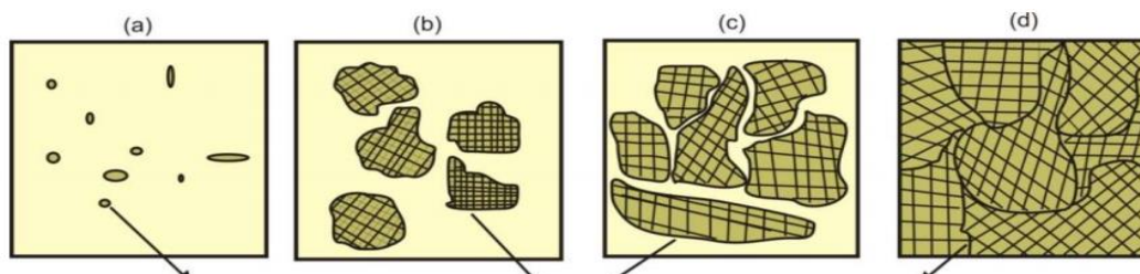
Slika 36. Shematski prikaz skrućivanja metala: (a) nukleacija kristala u taljevini metala; (b) i (c) rast kristala s napredovanjem skrućivanja; (d) skrućivanje je završeno (vide se pojedine granice zrna) [3]
