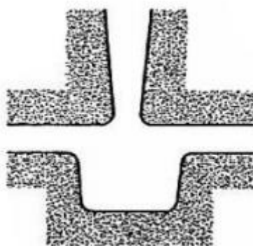
Slika 17. Oblikovanje razdjelnika [8]
