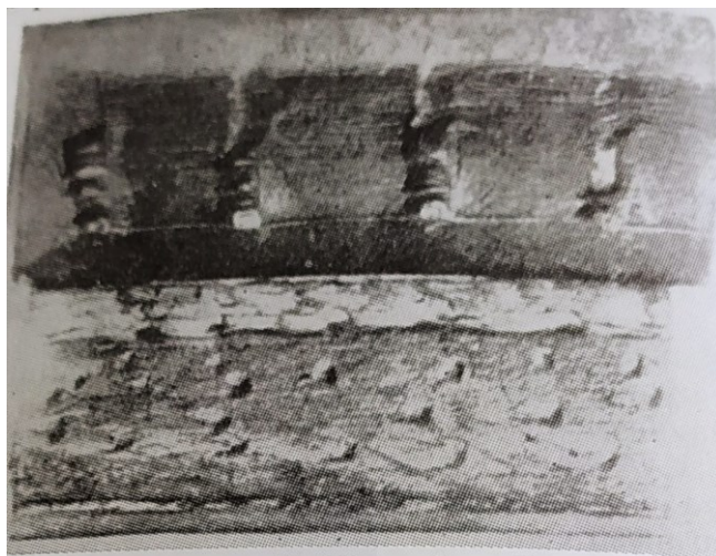
Slika 37. Greške nastale valjanjem na nasječnim i navarenim valjcima [16]
