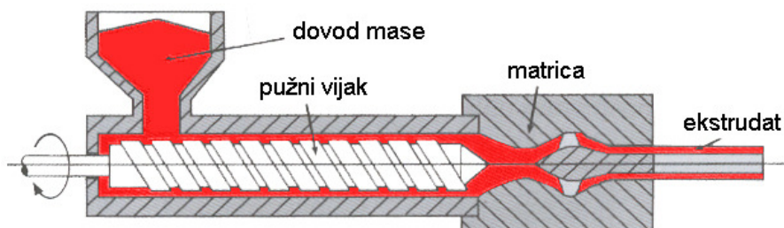
Slika 10. Ekstrudiranje [2]
