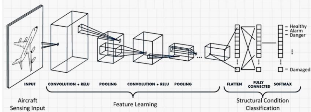
Slika 2.8. Prikaz uobičajene konvolucijske neuronske mreže [10]
