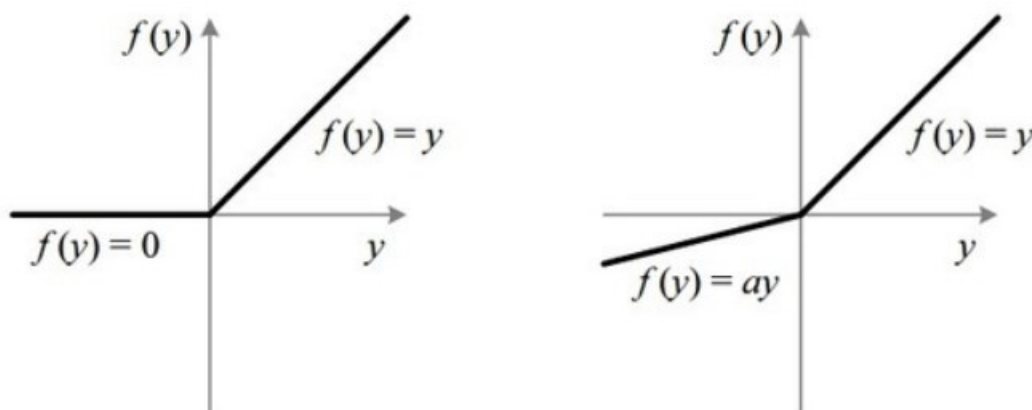
Slika 9. Obična ReLU (lijevo) i leaky ReLU (desno) funkcija.
