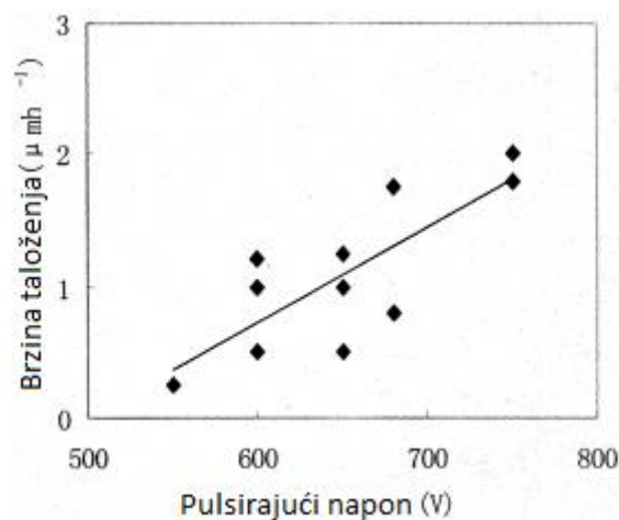
Slika 4.7 Brzina taloženja TiN prevlake u odnosu na visinu napona [20]
