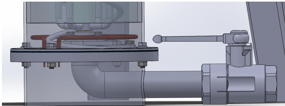
Slika 26. Ispust vode
