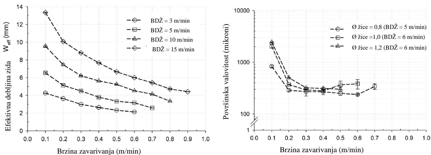
Slika 36. Ovisnost efektivne debljine zida o brzini zavarivanja (lijevo), ovisnost promjera žice o površinskoj valovitosti (desno) [20]
