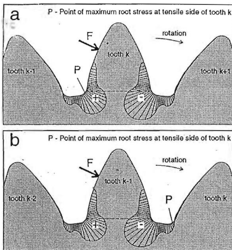
Slika 31. Naprežanje u korijenu zuba k u trenutku kada opterećenje djeluje na operativni bok promatranog zuba (a) i kada opterećenje djeluje na operativni bok zuba koji u zahvat ulazi nakon promatranog zuba (b) [13]
