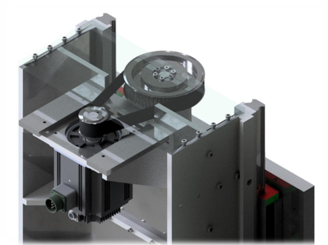
Slika 24. Pogon Z osi
