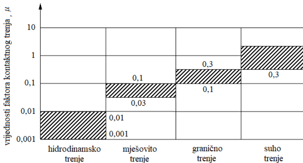
Slika 17. Rangiranje trenja prema Kloos-u [20]
