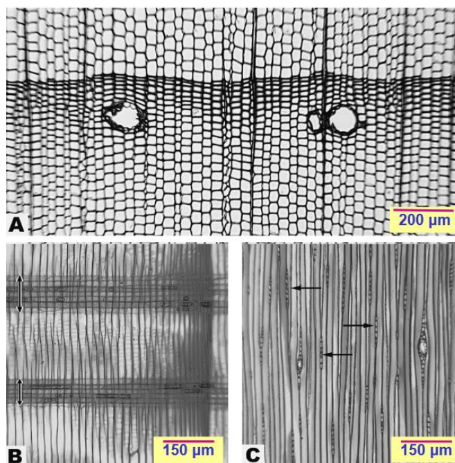
Slika 3. Karakteristični presjeci kroz četinjaču: A-poprečni, B-radijalni, C-tangencijalni [3]
