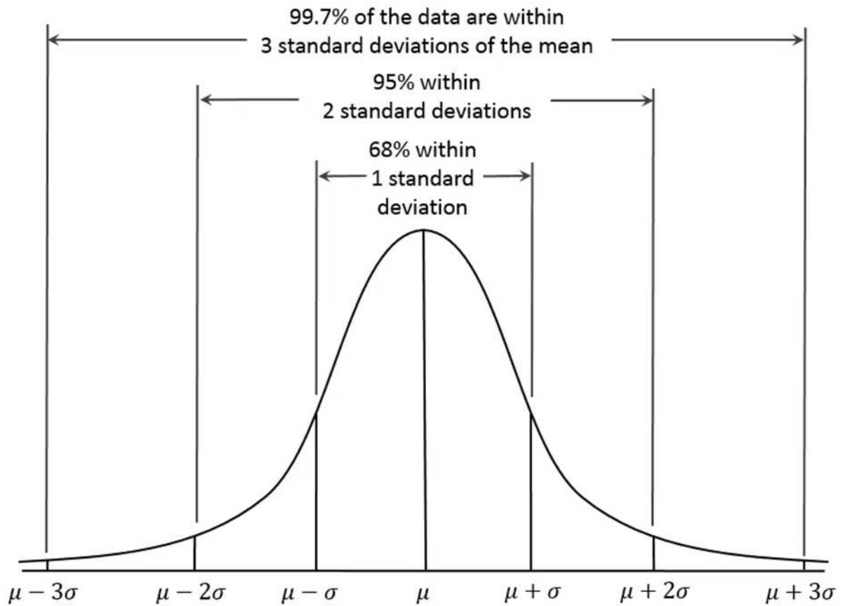
Slika 15. Normalna raspodjela
