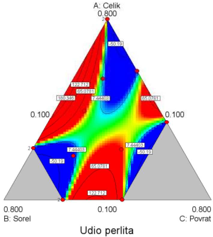
Slika 27 Dvdimenzionalni grafički prikaz dobivenog matematičkog modela za udio perlita
