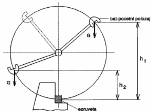
Slika 5.2. Mjerenje udarnog rada loma na Charpy-evom batu
