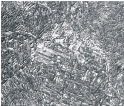
Maksimalna temperatura toplinskog ciklusa 1350 °C povećanje 100x povećanje 200x
