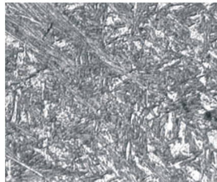
Maksimalna temperatura toplinskog ciklusa 1350 °C povećanje 100x povećanje 200x
