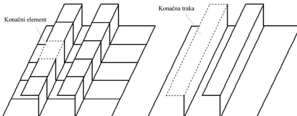
sl. 30 Diskretizirani model dijela orebrane tankostjene konstrukcije
