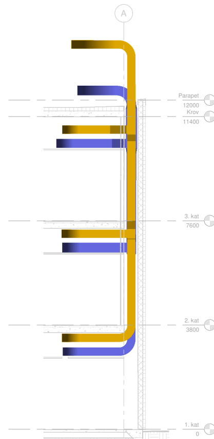
③ V_VO_3 1 : 50
