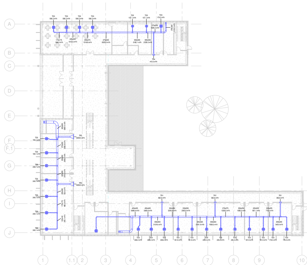
1 Dobavni sustav 1 : 200
