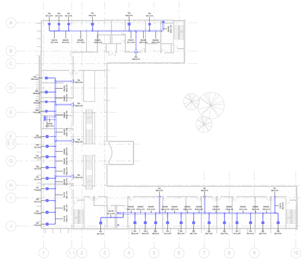
2 Dobavni sustav 1 : 200
