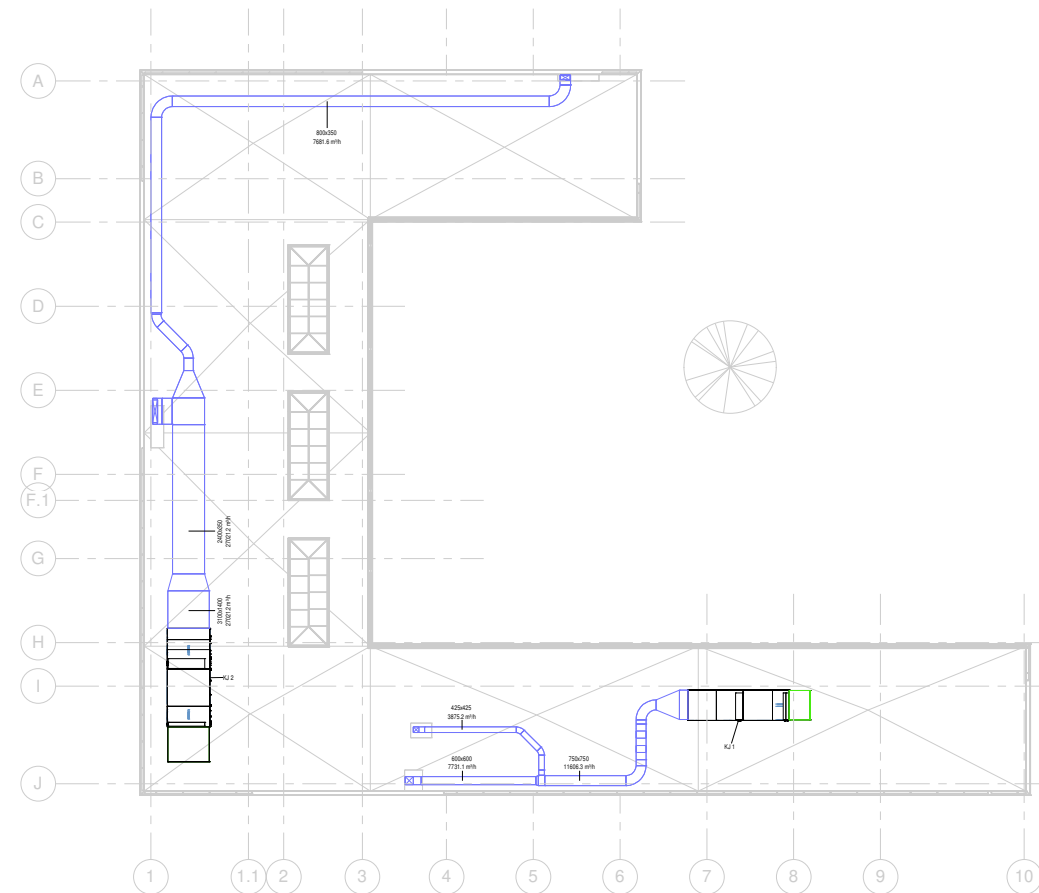
2 Dobavni sustav 1 : 200
