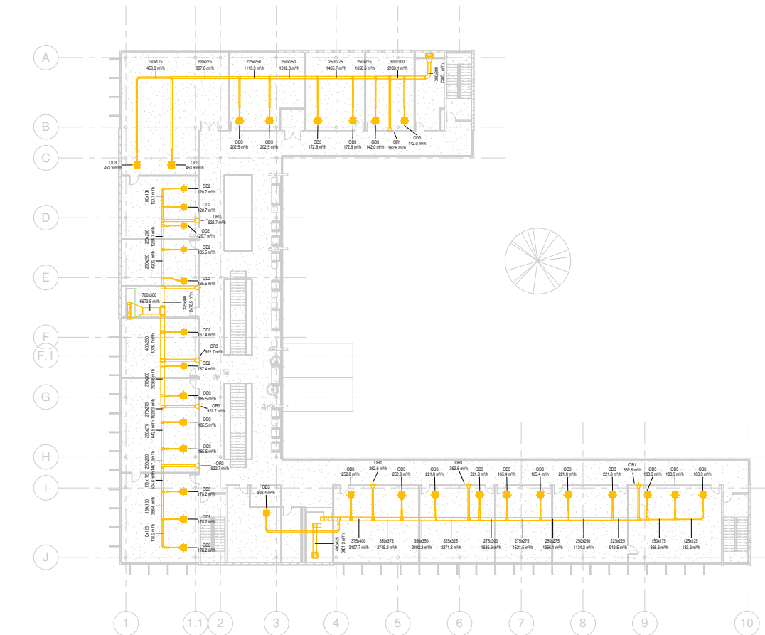
1 Odsisni sustav 1 : 200
