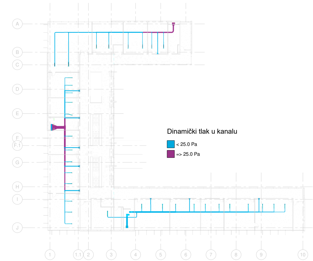
2 Odsisni sustav 1:200
