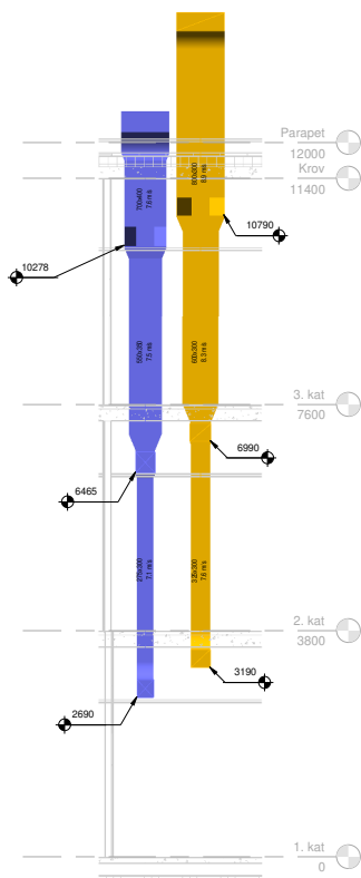
② H_VO_3 1 : 50
