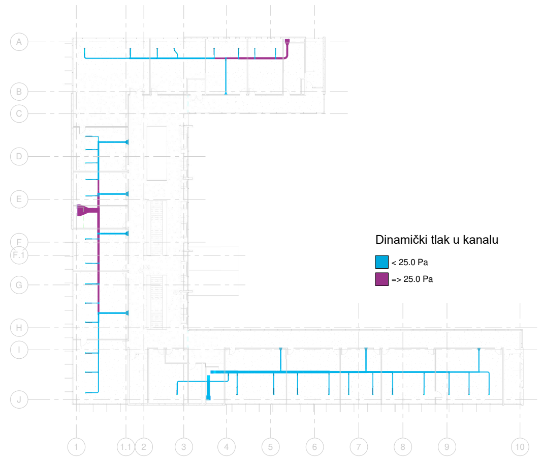
3 Dobavni sustav 1:200
