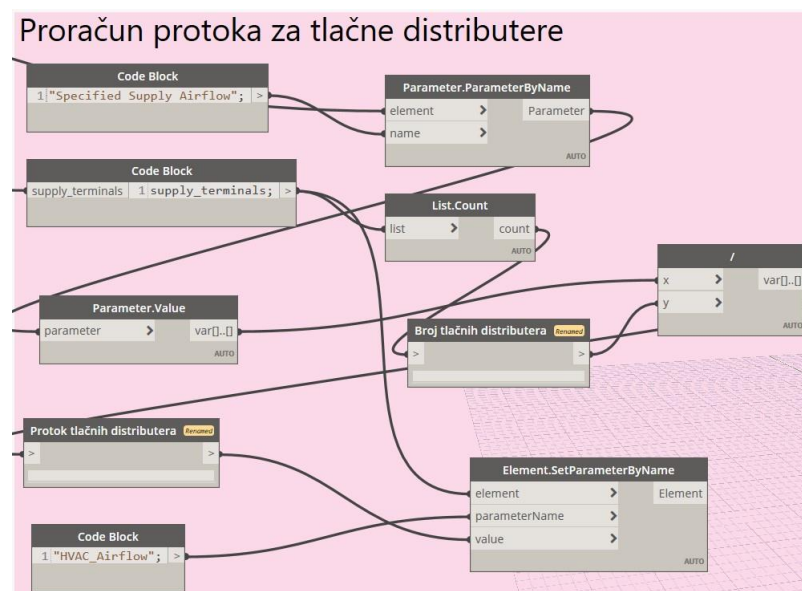
Slika 23 Proračun protoka distributera u prostoriji - 2. dio
