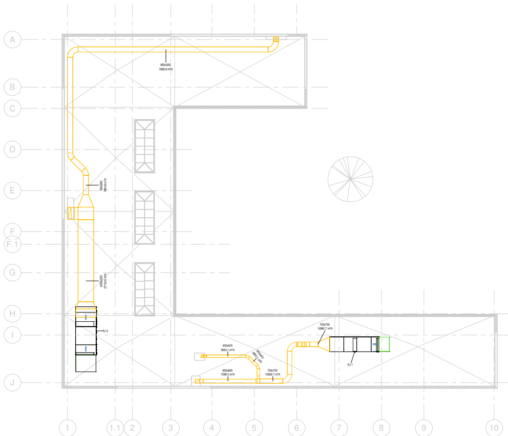
1 Odsisni sustav 1 : 200
