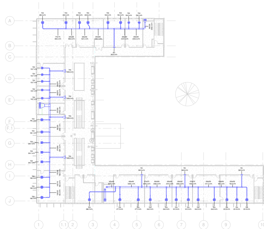
2 Dobavni sustav 1 : 200
