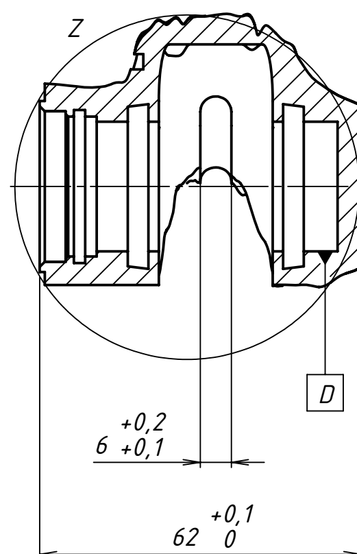
PRESJEK A-A
