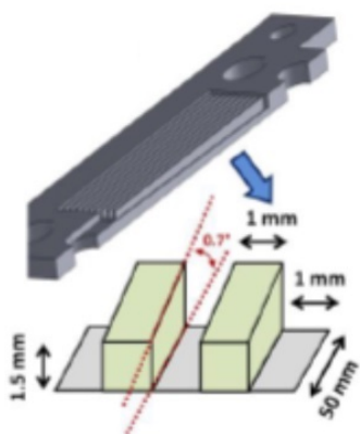
Slika 15. Klinasti oblik presjeka kanala [21]
