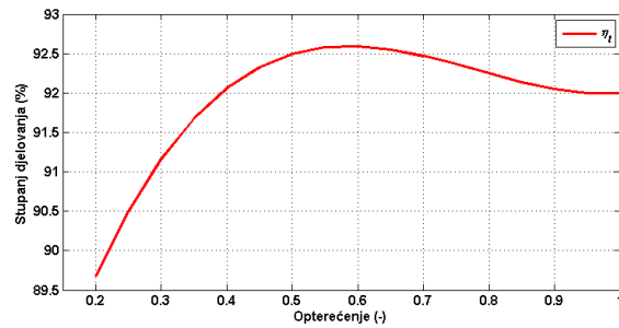
Slika 53. Prikaz ovisnosti stupnja djelovanja jedinice vrelodnog kotla o relativnom opterećenju
