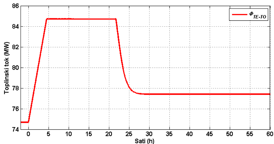
Slika 35. Predan toplinski tok s izvora toplinske energije (prag TE-TO ) u sustav Realnog modela pri konstantom dodatnom toplinskom toku od 10 \text{ MW}_t pri temperaturi okoliša od 0 \text{ }^\circ\text{C}
