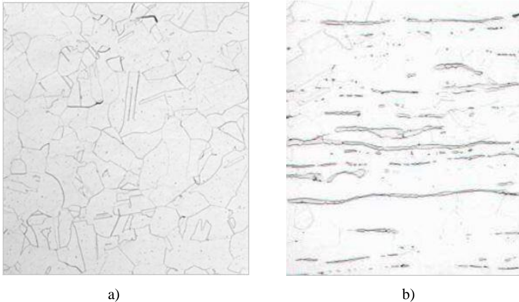
Slika 3. Mikrostruktura austenitnog nehrđajućeg čelika: a) 100% austenit; b) austenit i delta – ferit [12]
