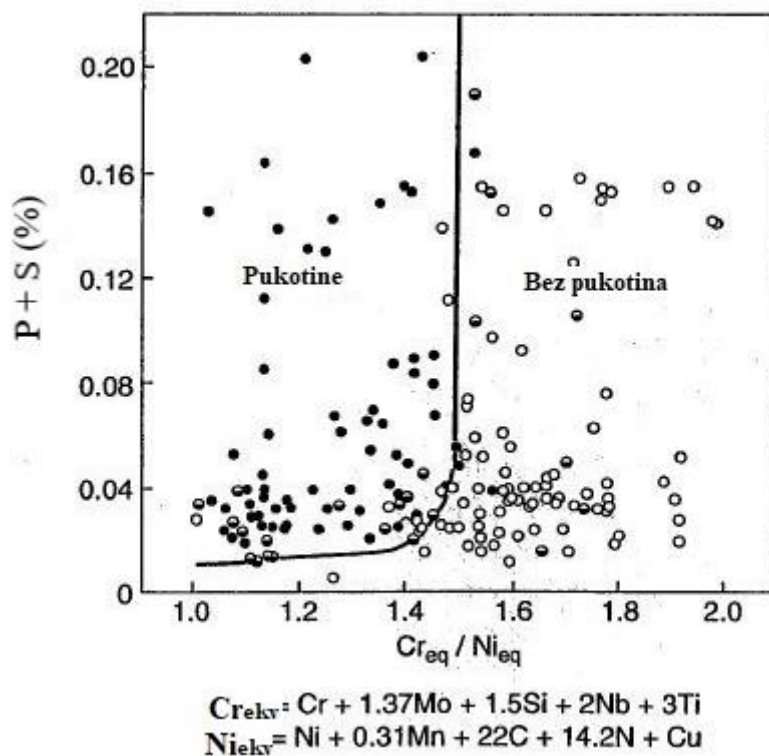
Slika 11. Suutala dijagram za predviđanje nastanka toplih pukotina [11]
