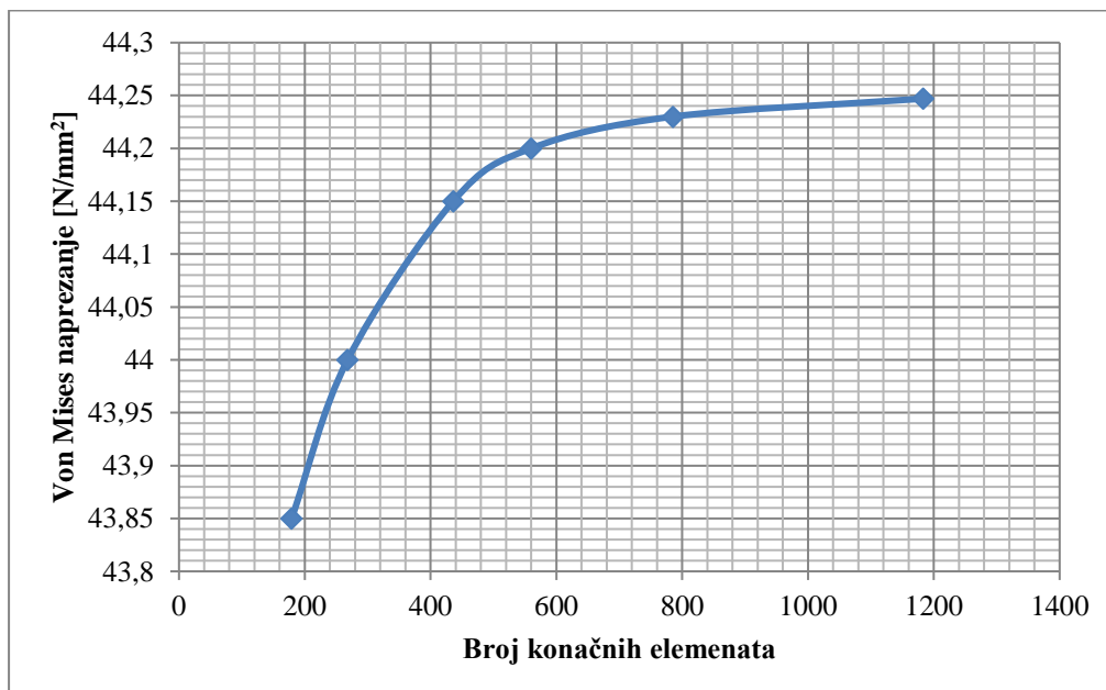
Slika 82. Konvergencija modela
