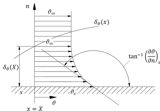
Slika 3.4. Temperaturni granični sloj fluida uz stijenku [6]
