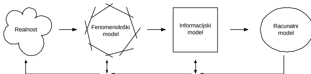
Slika 1: Preslikavanja od realnosti do racunalnog modela
