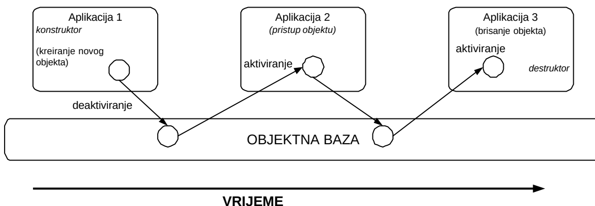
Slika 21: Proces aktiviranja i deaktiviranja objekata, prema [99]
