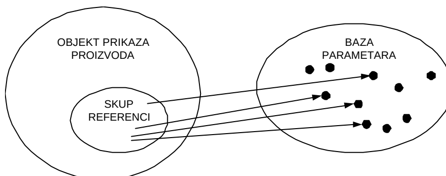
Slika 30: Skup referenci na parametre u bazi parametara kao podskup objekta prikaza proizvoda
