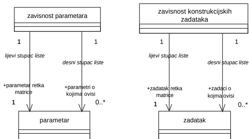
Slika 53: Matrice zavisnosti parametara i zadataka
