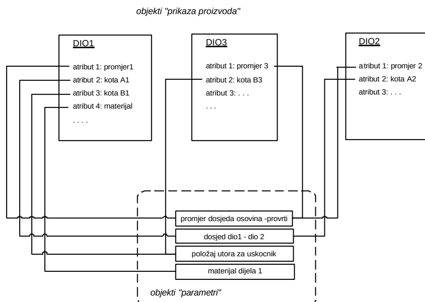
Slika 27: Povezivanje "zajedničkih" atributa objekata referenciranjem istog parametra
