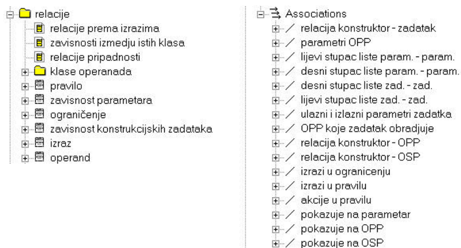
Slika 52: Klase i asocijacije u paketu "relacije"
