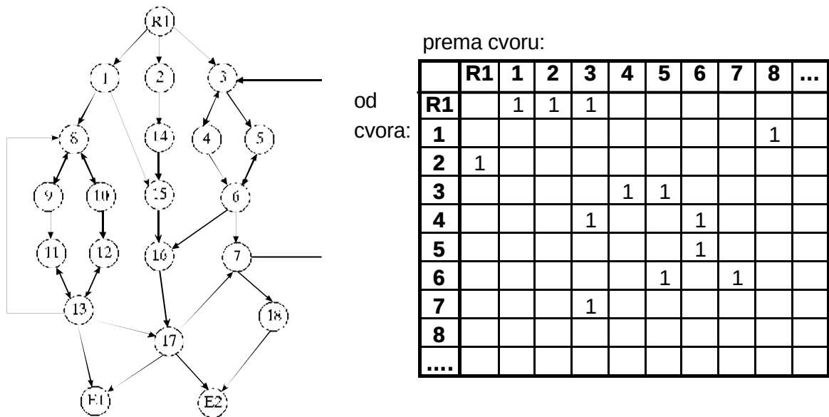
Slika 16: Usmjereni graf i dio njegove matrice susjedstva
