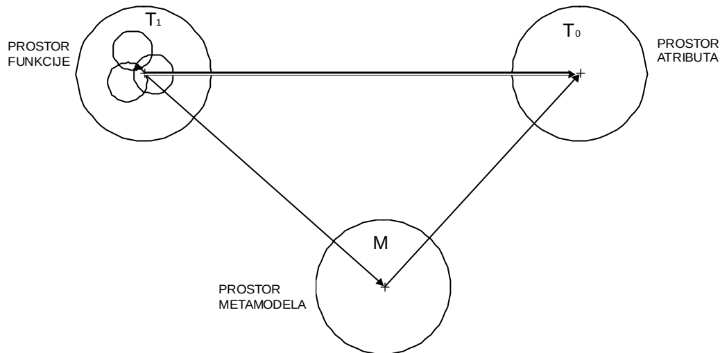
Slika 11: Koncept metamodela [70]
