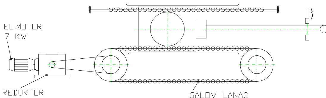
Slika 3.17. Funkcionalna shema potiska cijevi preko kolica [19]
