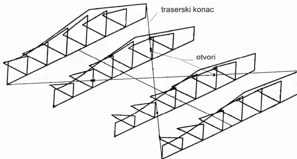
Slika 14: Kontrola prostornih dijagonala traserkim koncem
