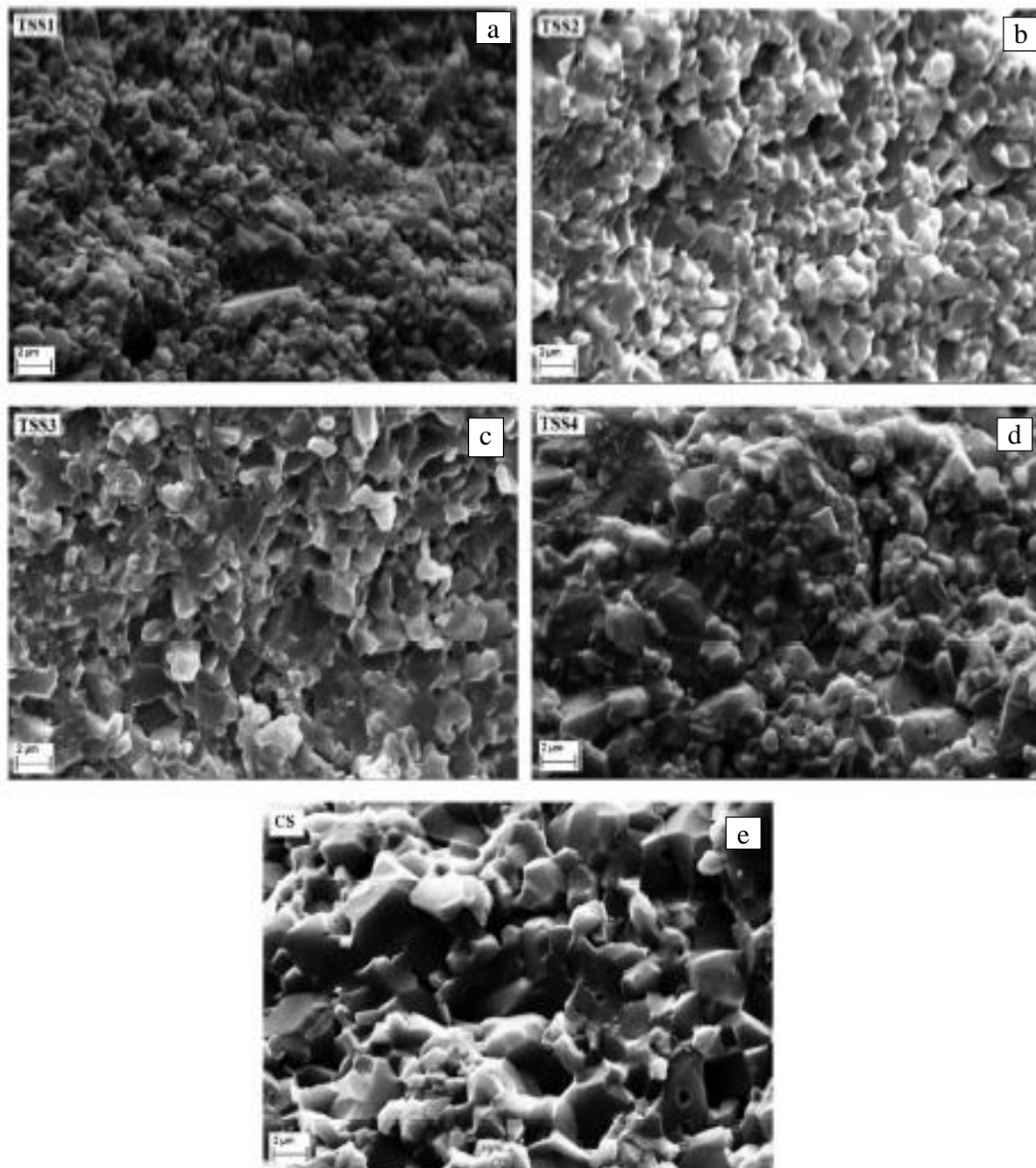
Slika 25. SEM fotografije mikrostrukture Al 2 O 3 keramike postignute (a, b, c, d) dvostupajskim sinteriranjem (TSS) i (e) konvencionalnim (CS) [37]
