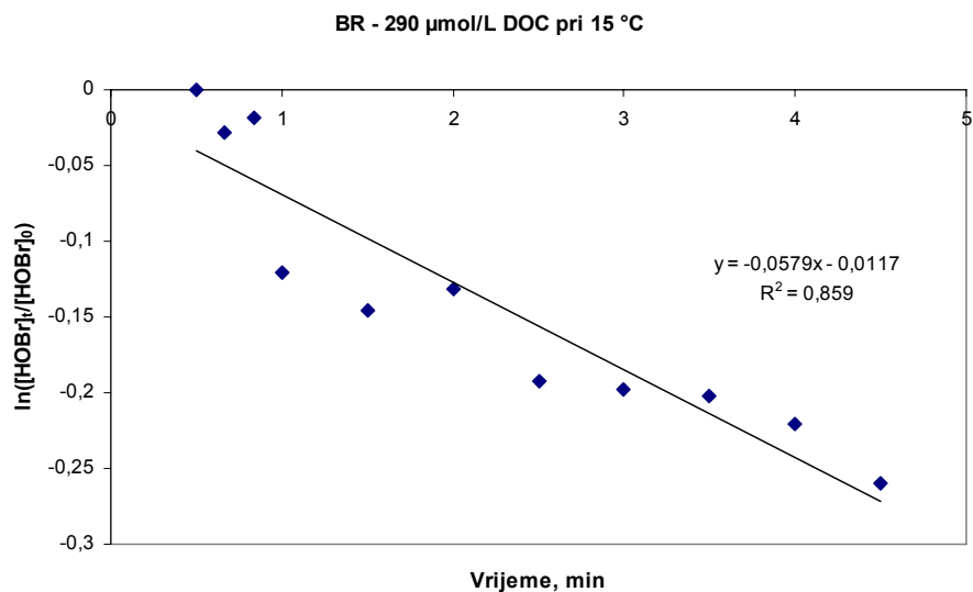
Slika 72. Kinetika raspada HOBr/OBr - pseudo prvog reda pri 15 °C i koncentraciji otopljenog organskog ugljika od 290 \mu\text{mol/L} površinske vode Black River
