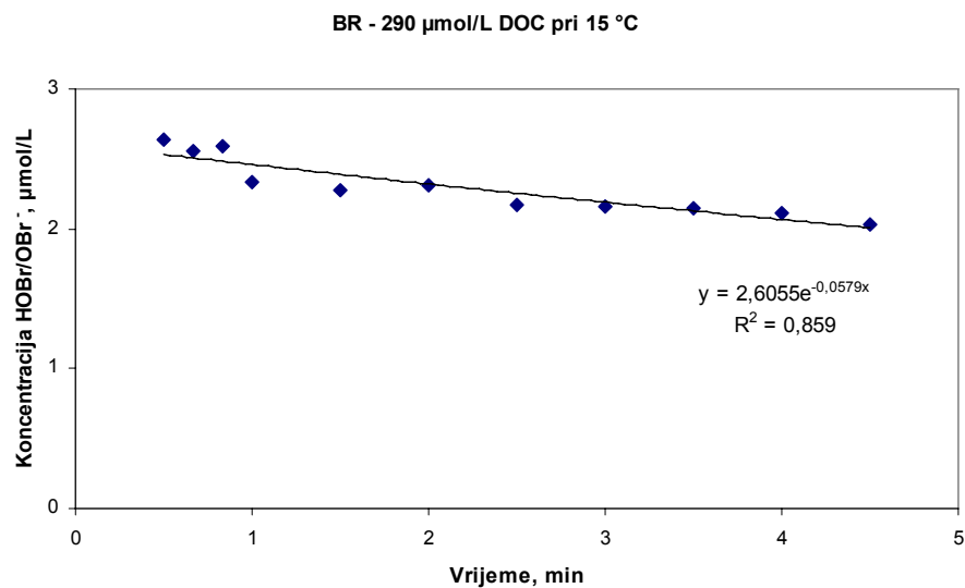
Slika 71. Raspad HOBr/OBr - u mraku pri 15 °C i koncentraciji otopljenog organskog ugljika od 290 \mu\text{mol/L} površinske vode Black River
