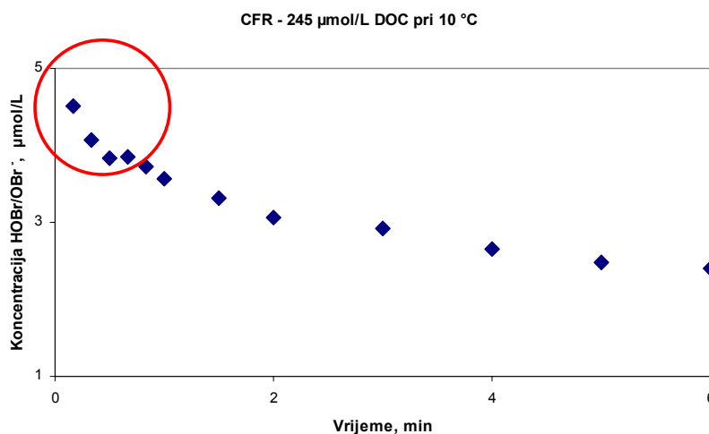
Slika 106. Kinetika raspada ukupnog raspoloživog broma s naznačenom inicijalnom brzo potrošnjom broma u reakciji s prirodnim organskim tvarima pri 10 °C u površinskoj vodi Cape Fear River
