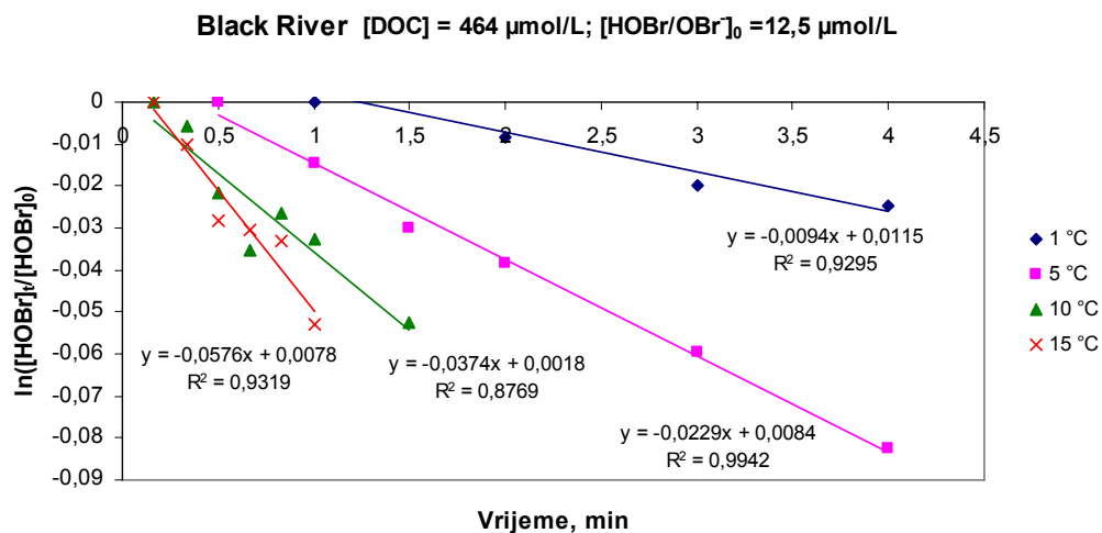
Slika 79. Sumarni prikaz konstanta brzine reakcije pseudo prvog reda slobodnog raspoloživog broma inicijalne koncentracije 12,5 \mu\text{mol/L} s otopljenim organskim ugljikom koncentracije 464 \mu\text{mol/L} površinske vode Black River
