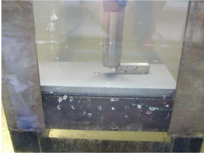
Slika 3.16 Etalon za određivanje slobodnog kraja žice pri zavarivanju Implant uzorka praškom punjenom žicom u plinskoj zaštiti
