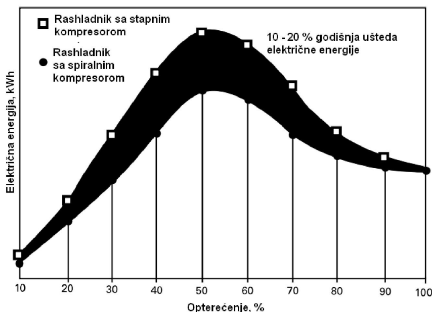
Slika 22. Ušteda električne energije rotacijskog kompresora u odnosu na stapne kompresore [10]
