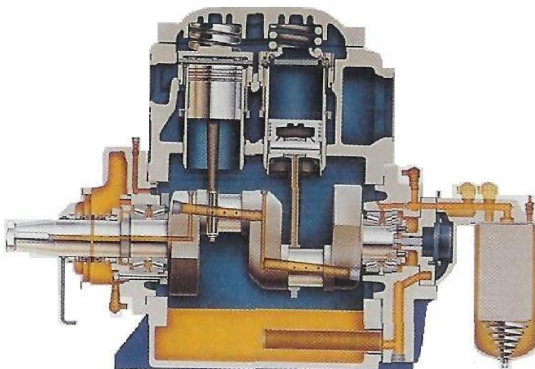
Slika 16. Stapni kompresor
