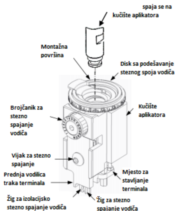
Slika 24. Dijelovi aplikatora [27]
