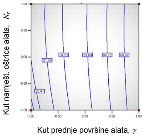
Slika 6.7. Hrapavost ovisna o kutovima \gamma i \chi_r
