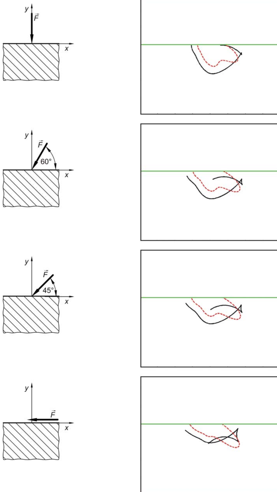
Slika 4.15 Simulacije krivulja kaustike i inicijalnih krivulja za različite uvjete opterećenja (CFRP131, \vartheta=45^\circ ).
