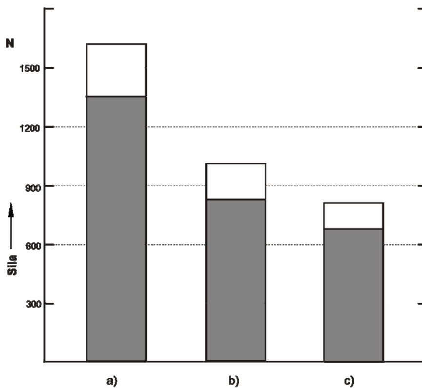
Slika 6.2 Kritična sila opterećenja CFRP131 kompozita za a) \varphi=90^\circ , b) \varphi=0^\circ i c) \varphi=45^\circ
