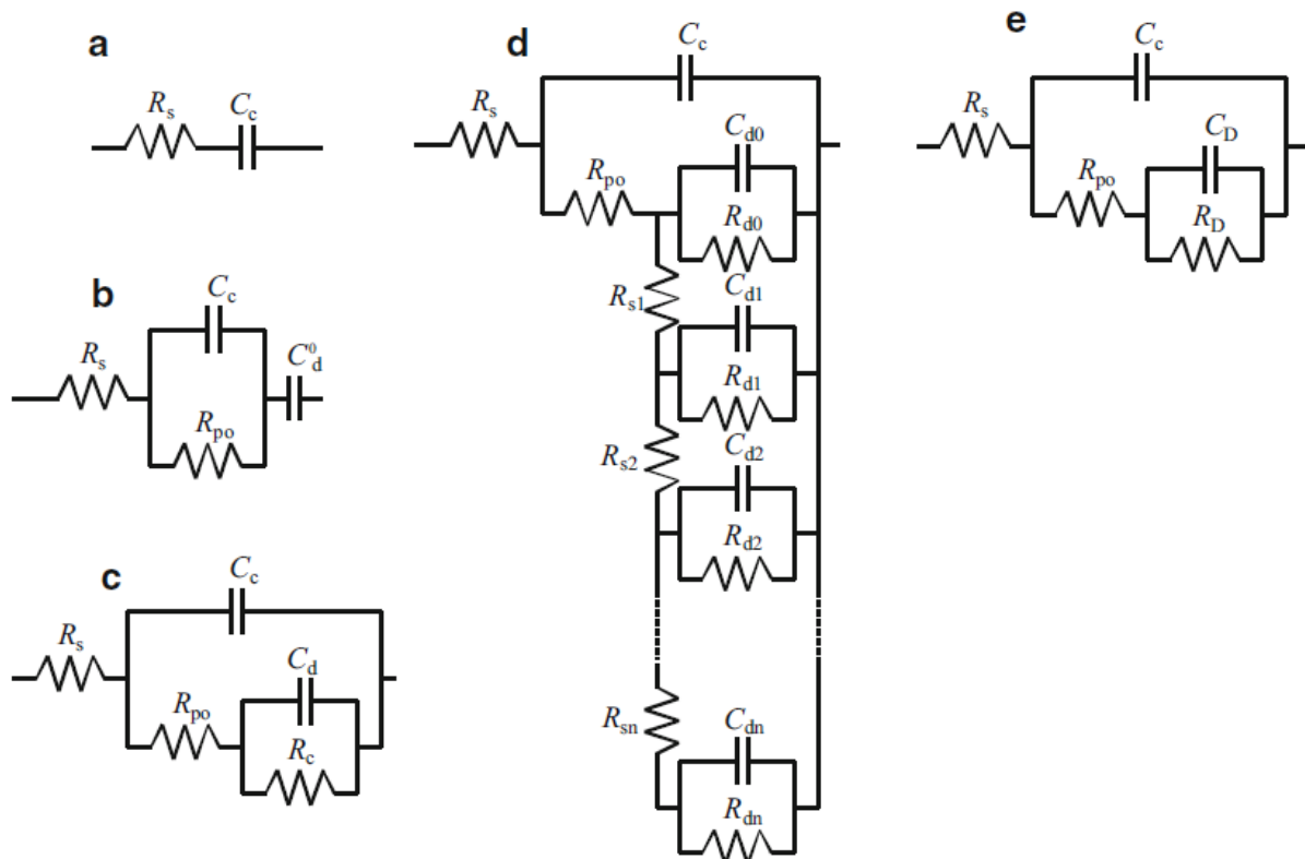
Slika 4.3. Električni ekvivalentni krugovi za organske prevlake [19]
