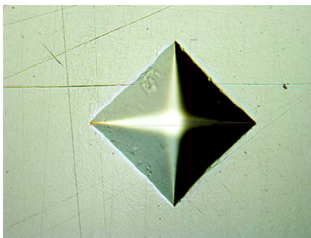
Slika 5.17: Prikaz otiska na opto-elektrničnom sustavu CCD-LFSB
