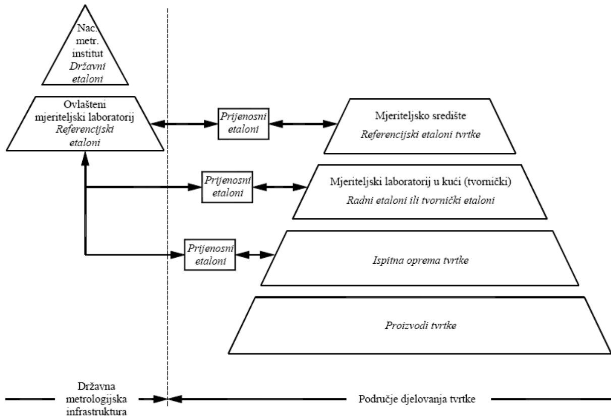
Slika 3.10: Hijerarhija umjeravanja [31]
