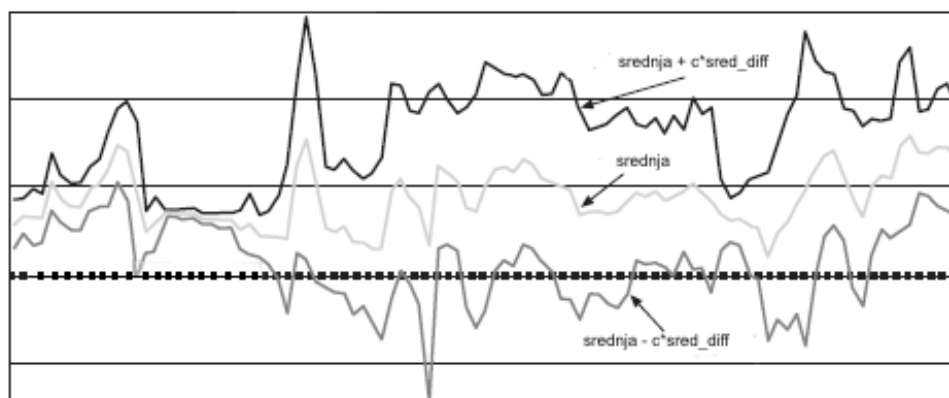
Slika 3-1 Segmentacija
