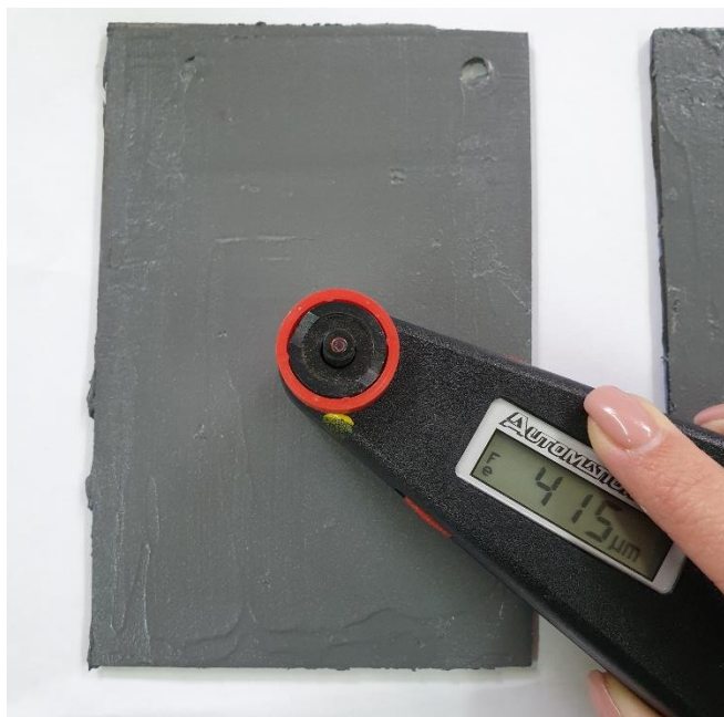
Slika 7.23. Mjerenje debljine filma premaza pomoću uređaja QuaNix 1500
