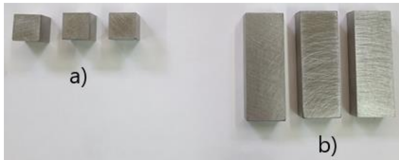
Slika 7.3. Nahrpavljeni uzorci prije nanošenja premaza: a) uzorci za ispitivanje na eroziju, b) uzorci za ispitivanje na abraziju
