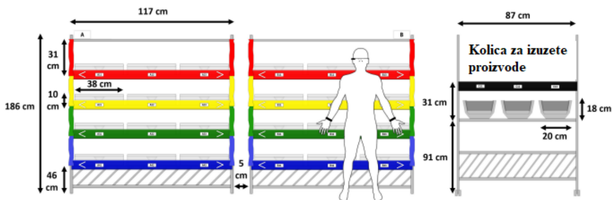
Slika 27. Eksperimentalno okruženje [14]
