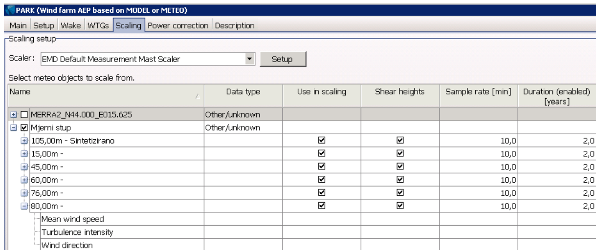
Slika 7.26: Odabir mjernih podataka u PARK modulu [28]
