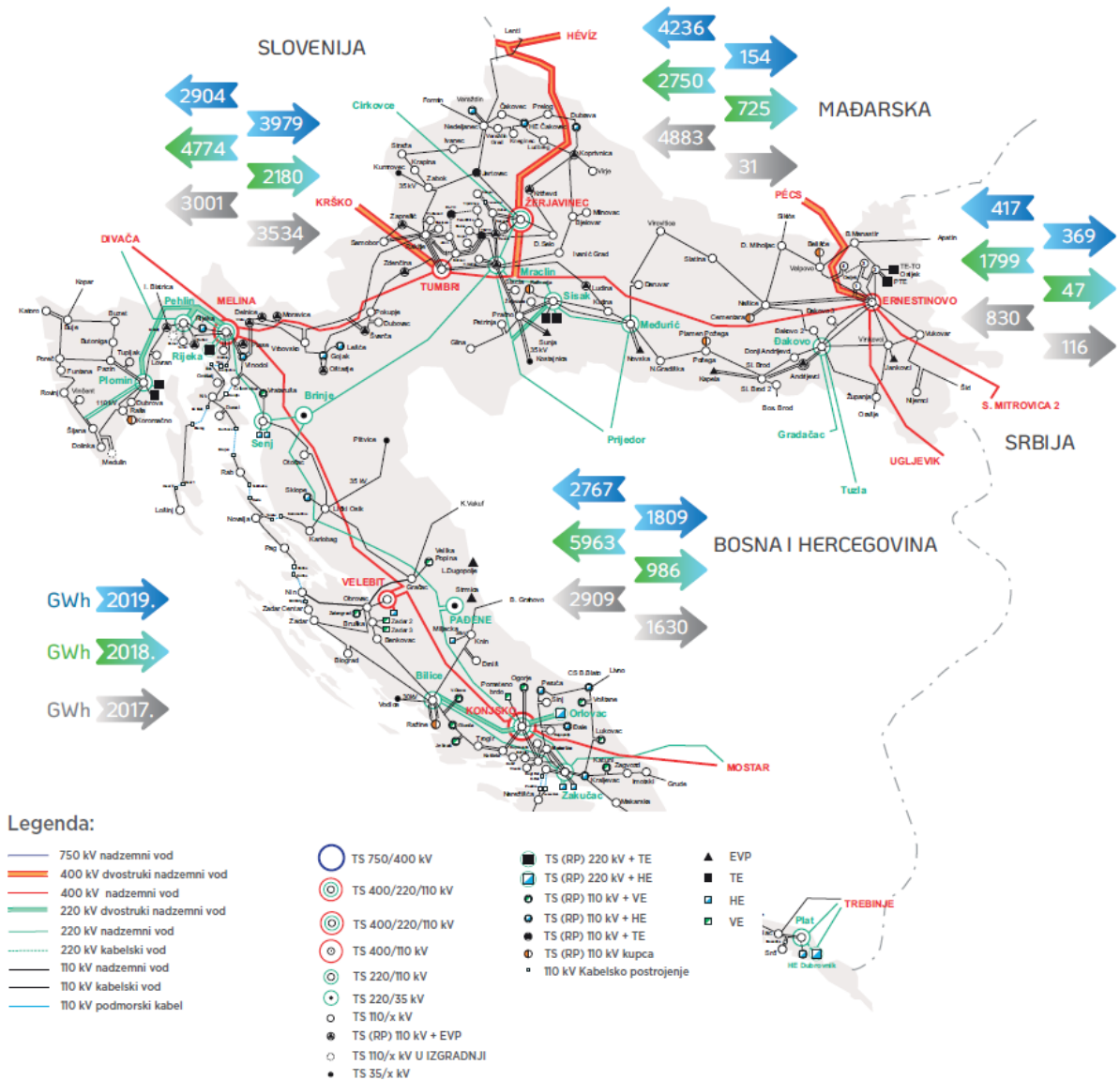
Slika 3.1: Prijenosna mreža Hrvatske i prekogranična razmjena energije [9]
