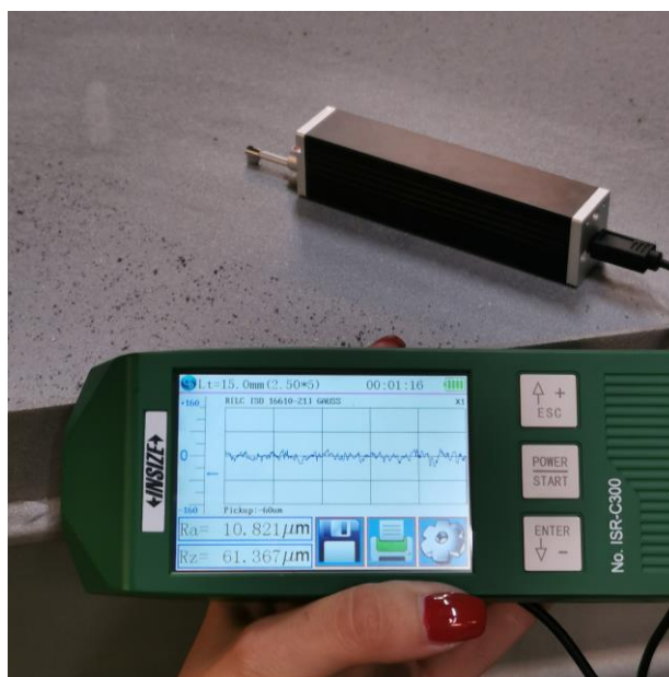
Slika 15. Mjerenje hrapavosti
